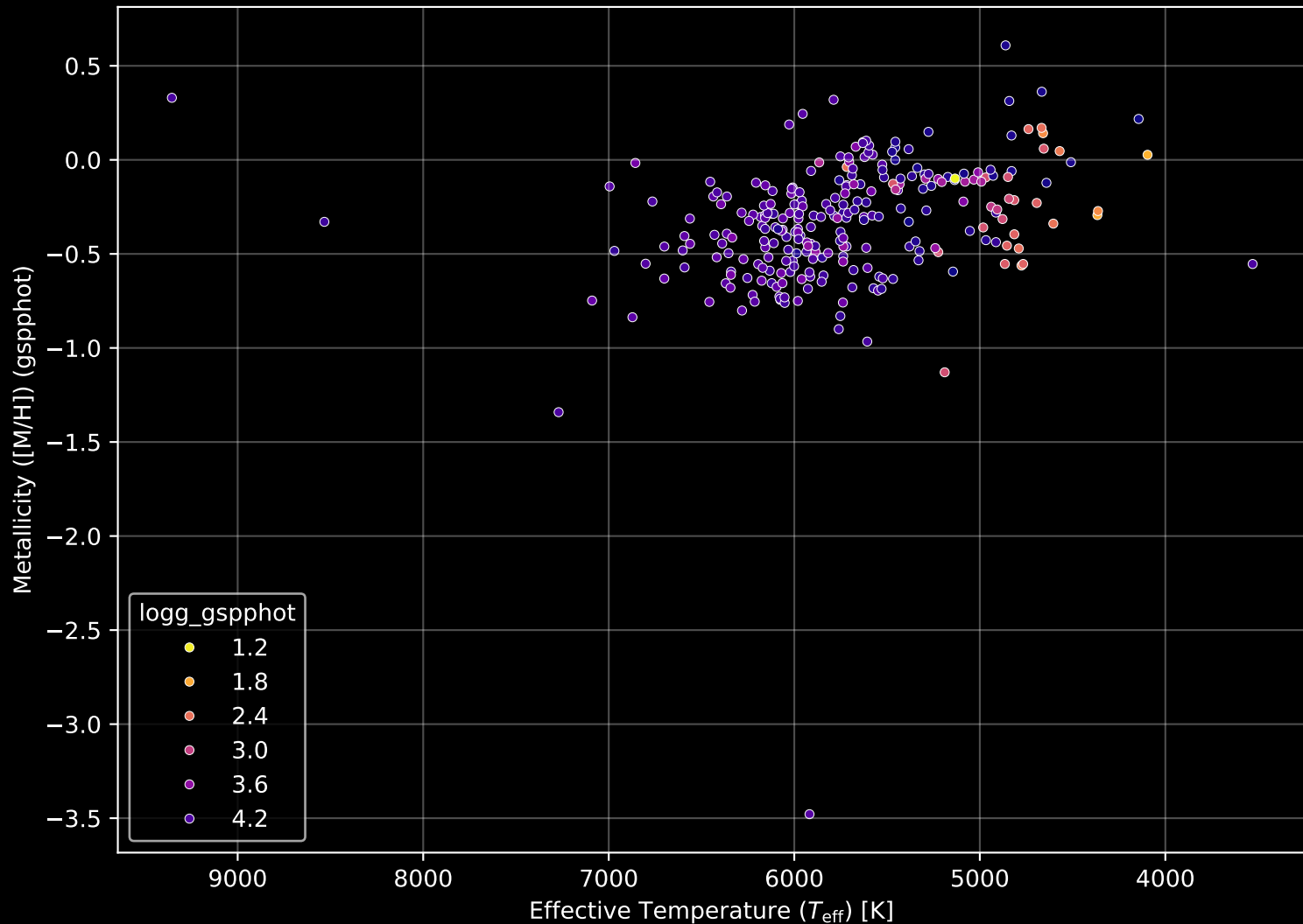
GALAH DR4 Field: [1615] Stellar Population Parameters (n= 264)
