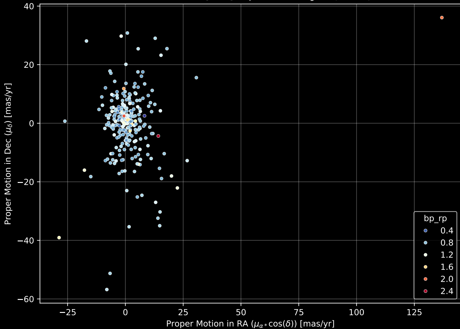
GALAH DR4 Field: [1615] Proper Motion Diagram (n= 264)
