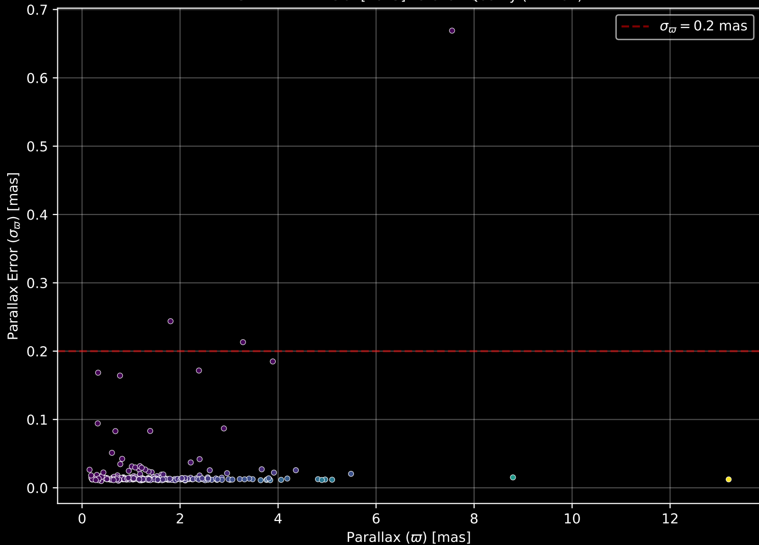
GALAH DR4 Field: [1615] Parallax Quality (n= 264)
