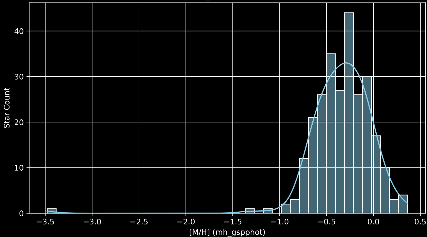
GALAH DR4 Field: [1615] [M/H] (mh_gspphot) (n= 263)
